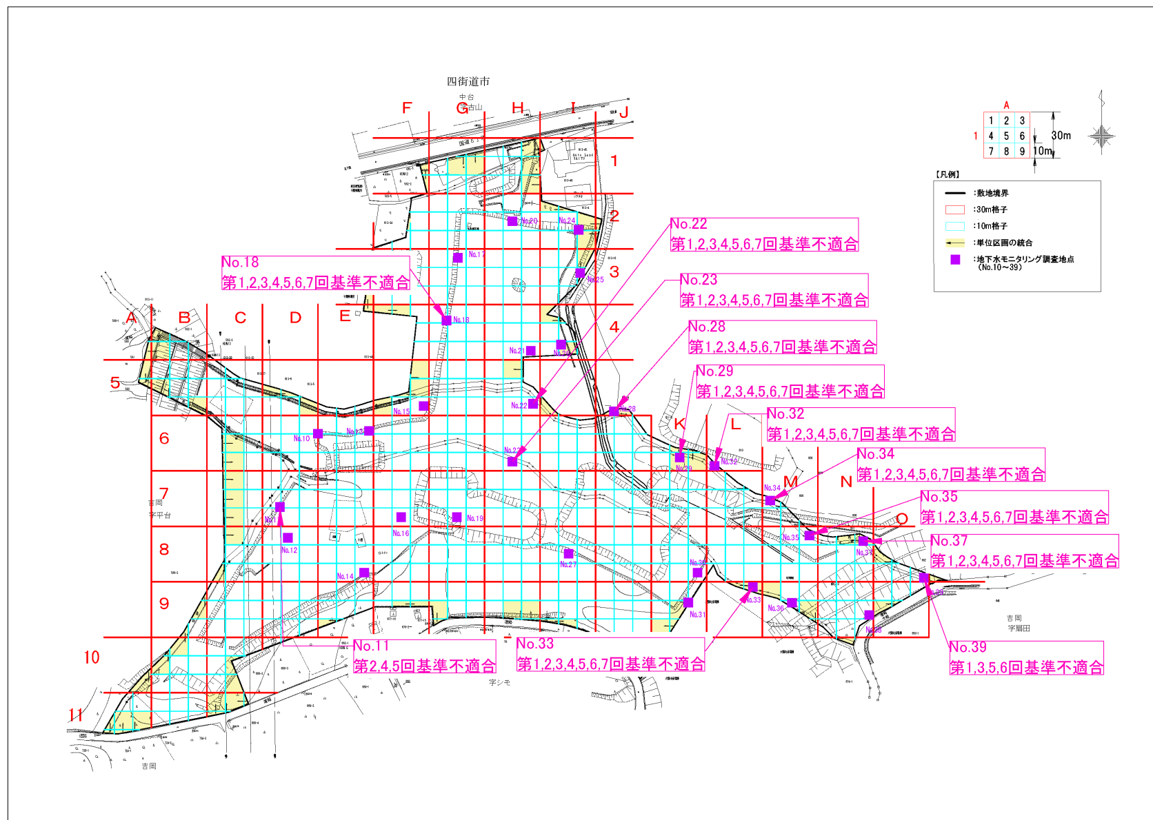
図 2-23 基準不適合地点(水素イオン濃度)
