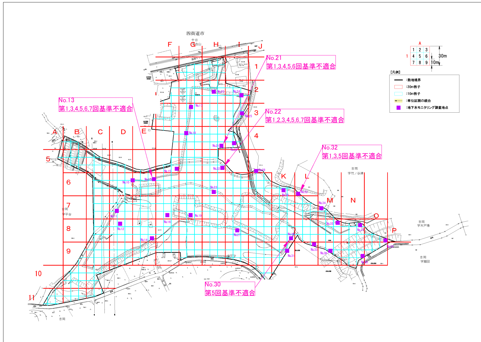
図 2-22 地下水基準不適合地点(ふっ素及びその化合物)
