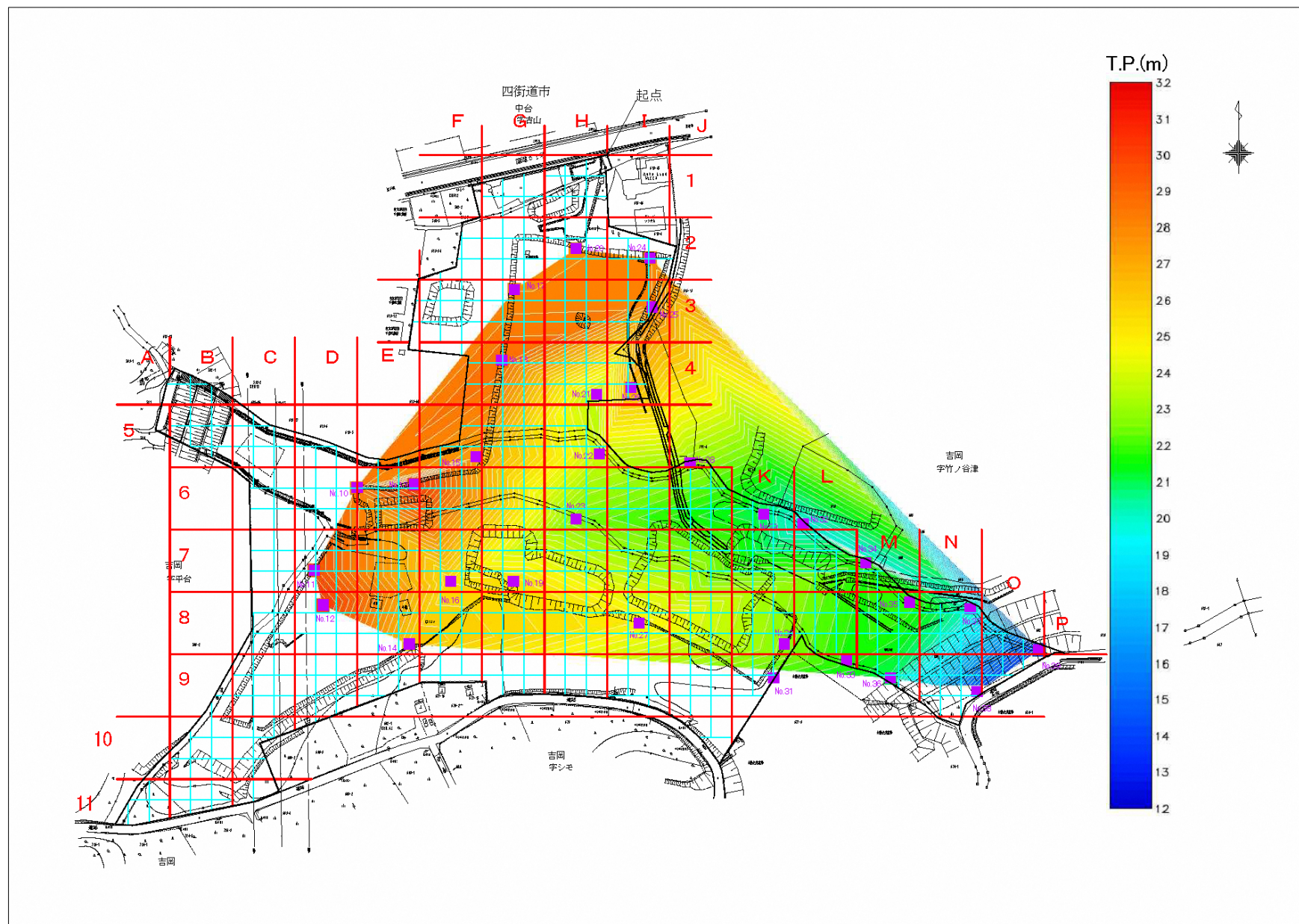
図 2-15 地下水位コンター図(1回目)
