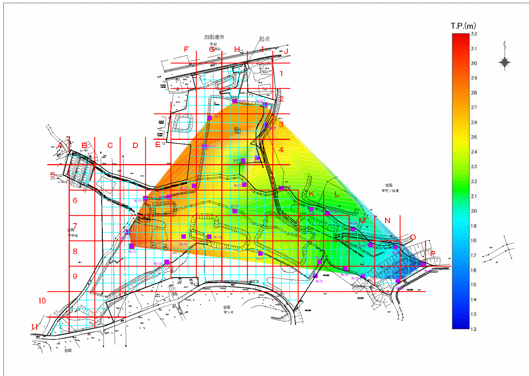
図 2-20 地下水コンター図(6 回目)
