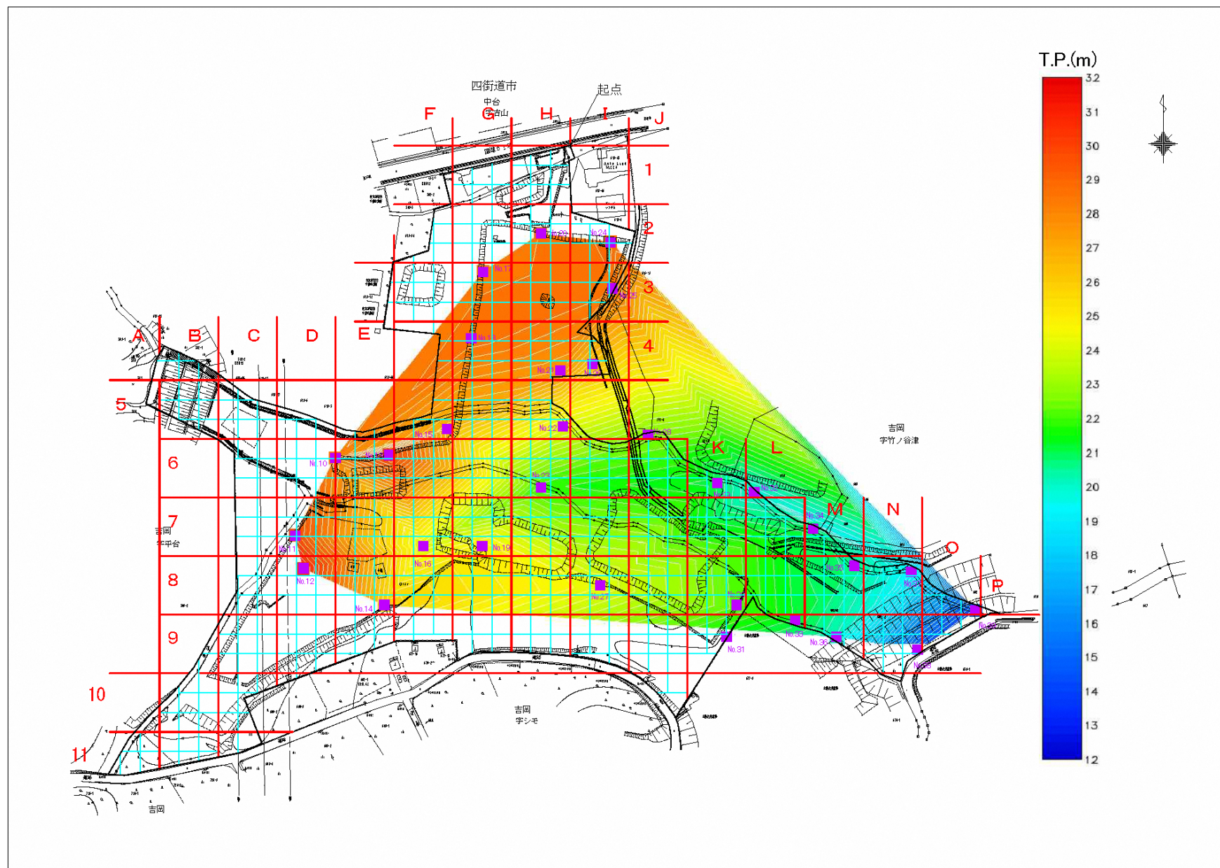
図 2-17 地下水位コンター図(3回目)
