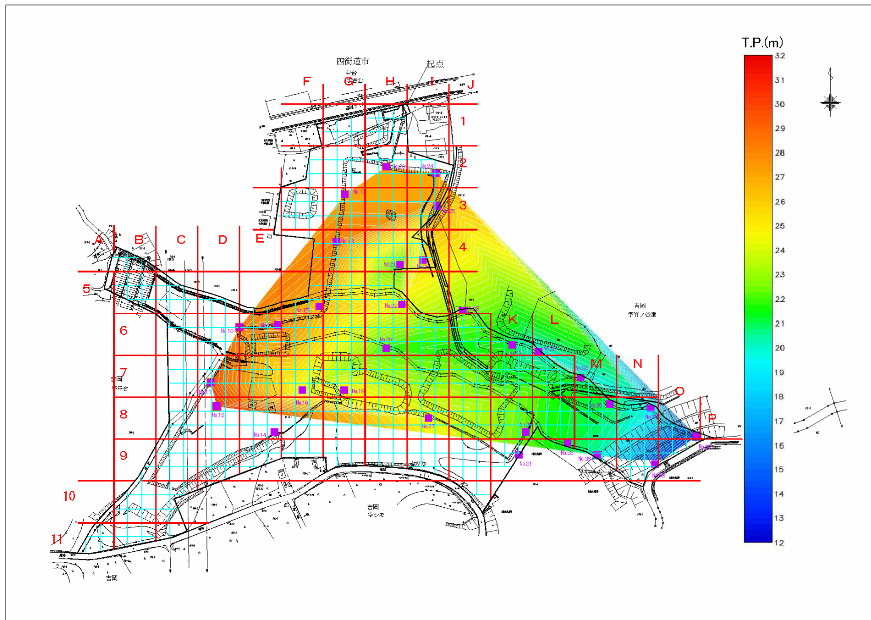
図 2-16 地下水位コンター図(2回目)
