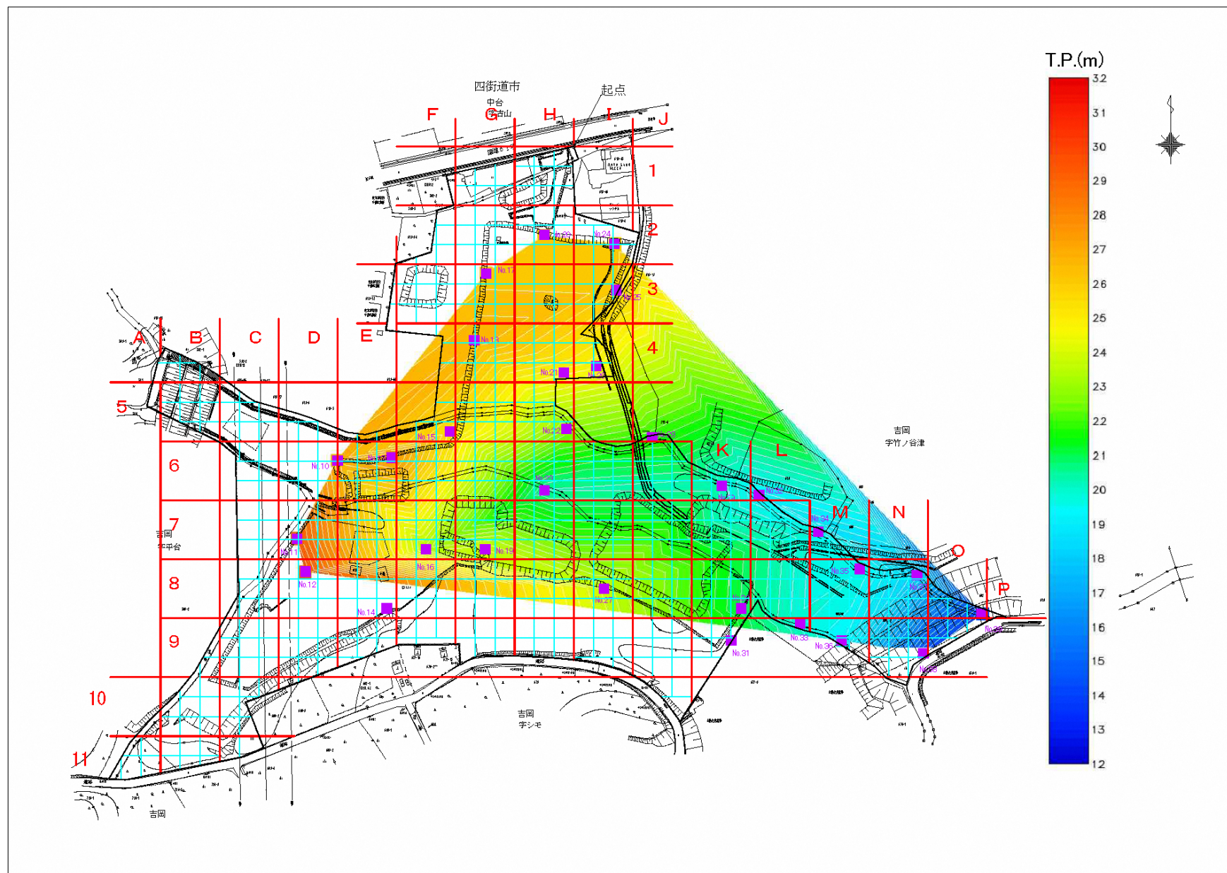
図 2-21 地下水コンター図(7 回目)
