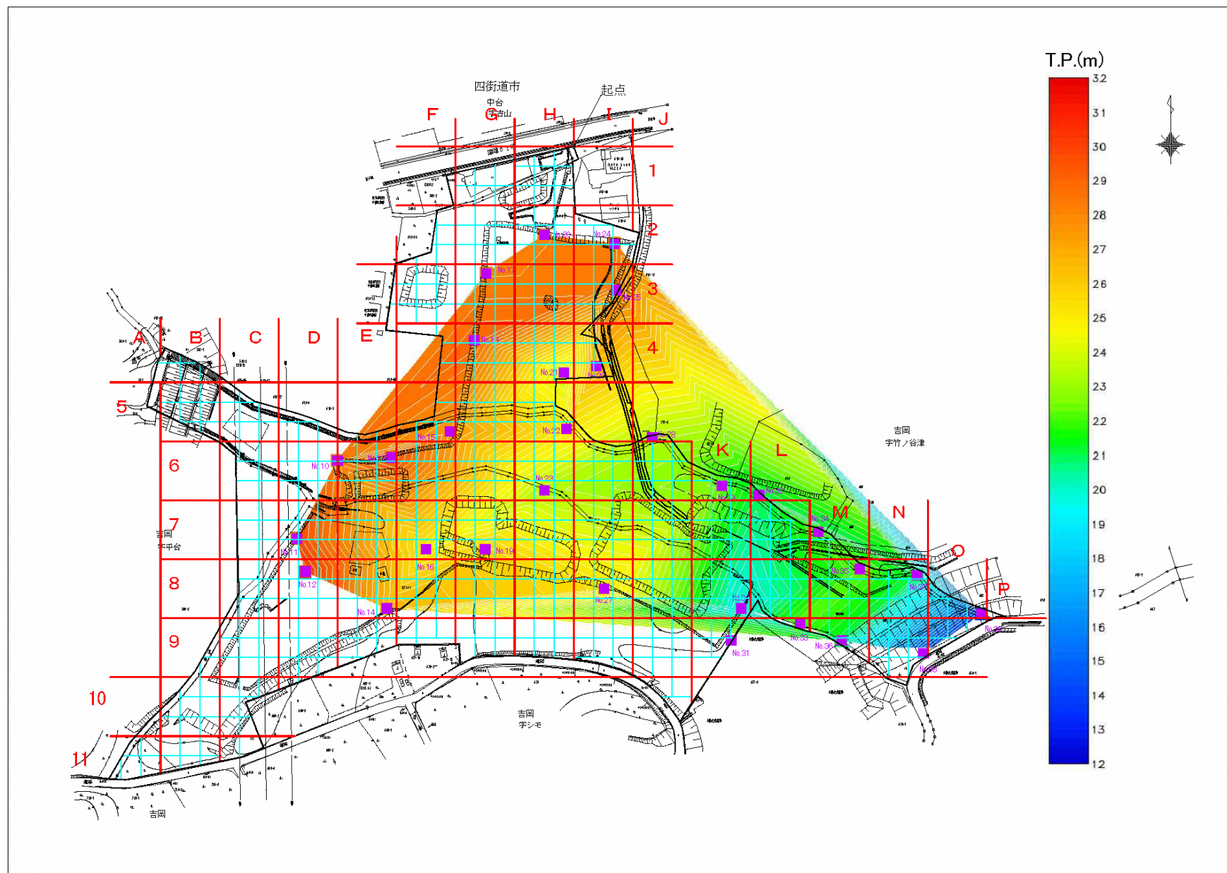
図 2-19 地下水位コンター図(5 回目)
