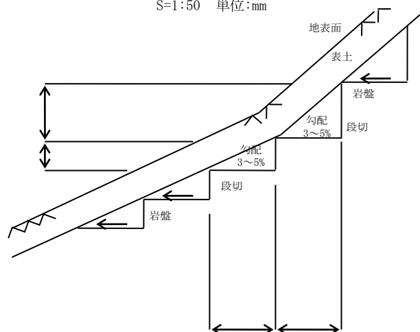
段切施工仕様図
