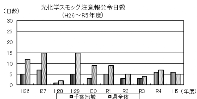
図表3-2-3 千葉地域における注意報の発令状況
