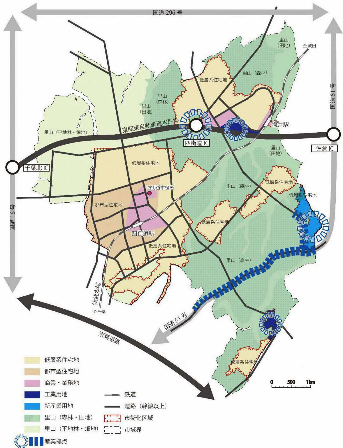
土地利用の方針図
