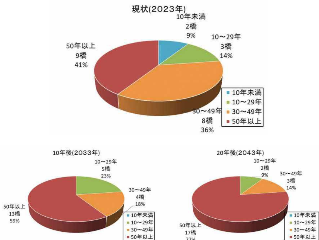
図 1-1 橋齢の推移
